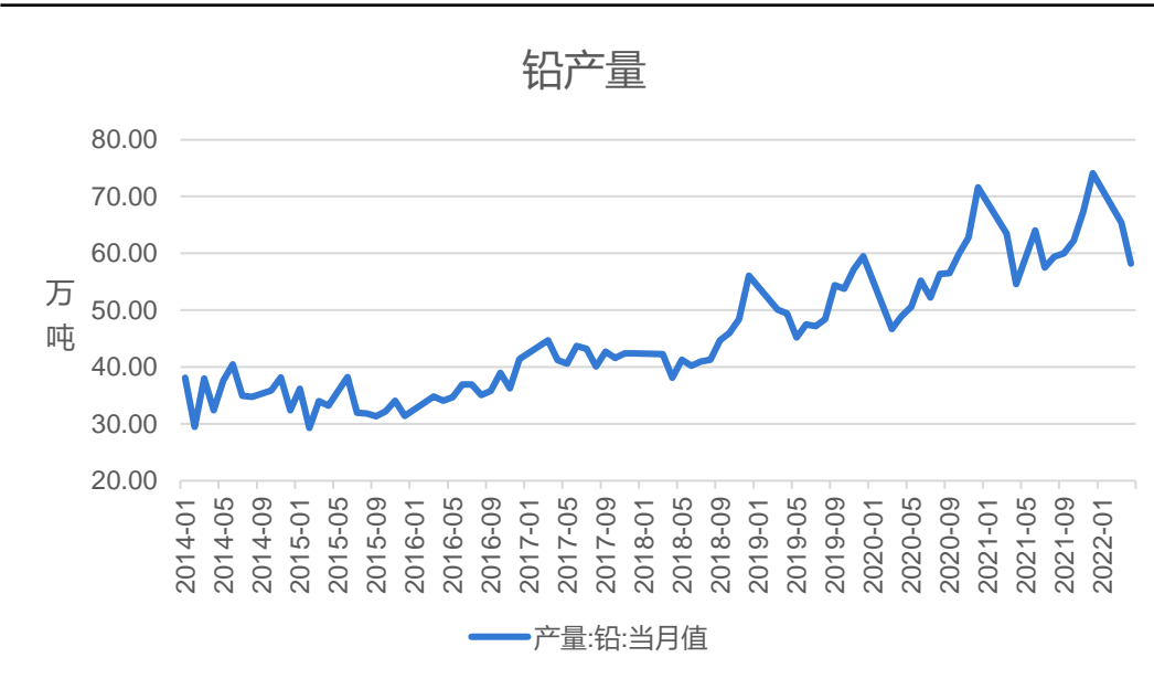
图14、铅产量
