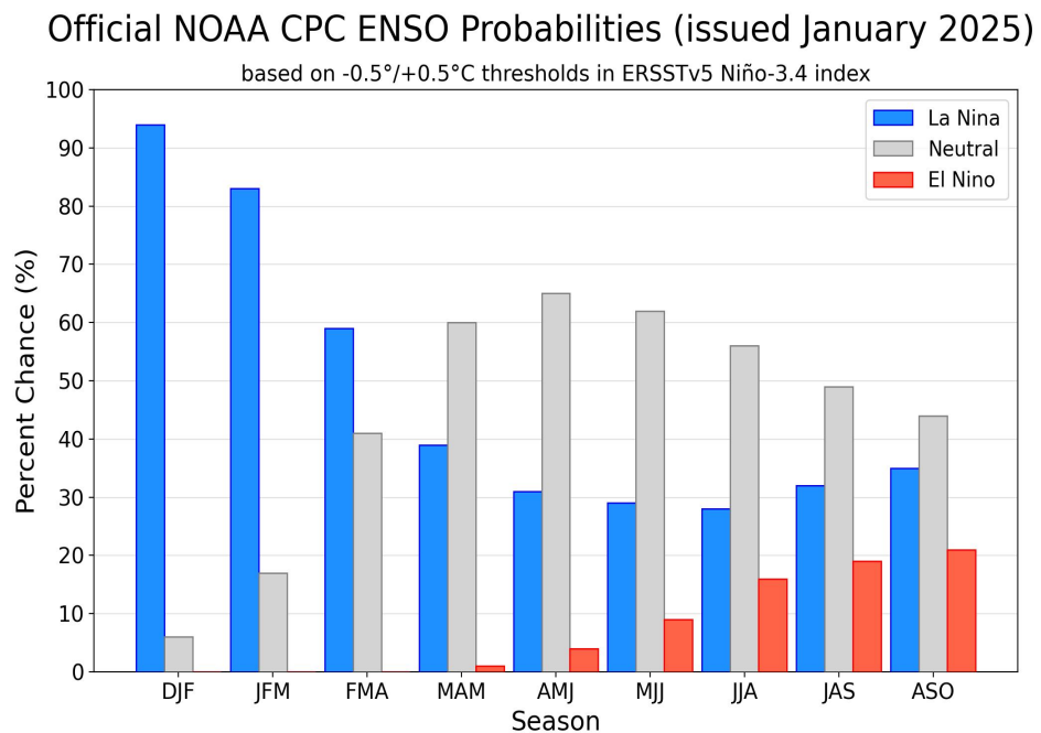
图 ENSO预测（1月）
