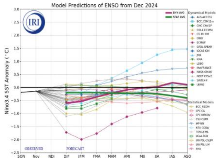
图 不同模型对ENSO指数的预测（1月）
