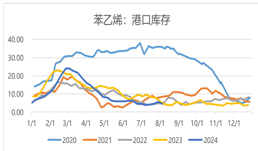
图31、苯乙烯港口库存
