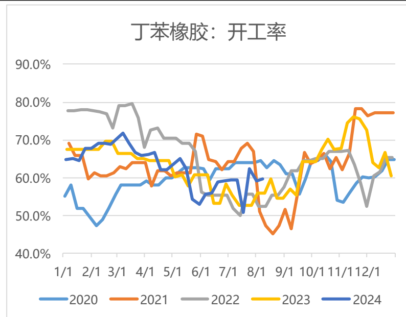
图20、丁苯橡胶开工率
