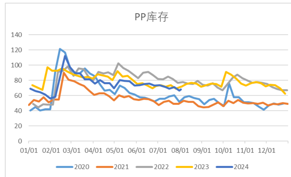
图19、PP库存
