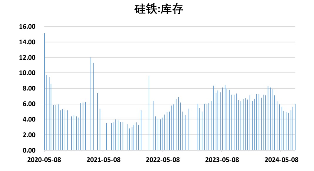
图10、硅铁库存
