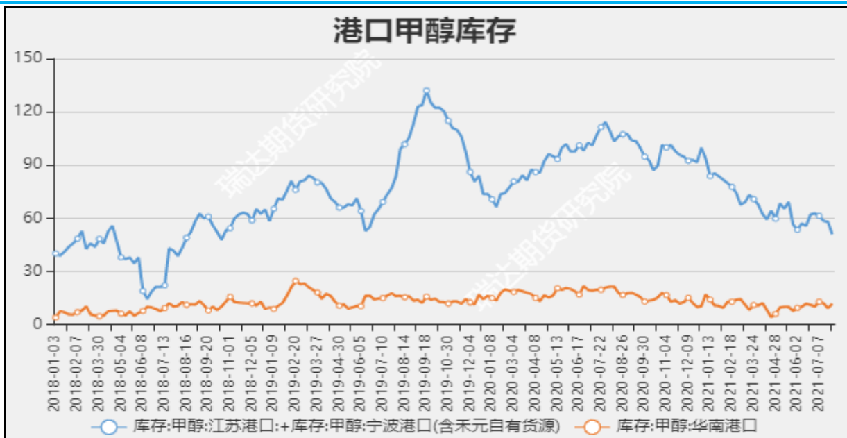
图11 甲醇港口库存
