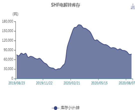
图13: 上海锌库存走势图
