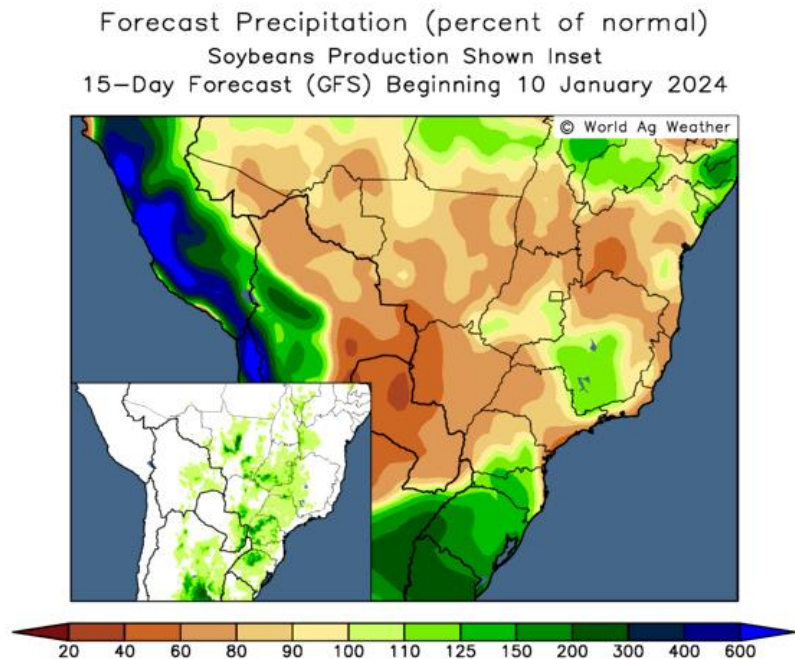
图 巴西未来15天降水距平 (%)
