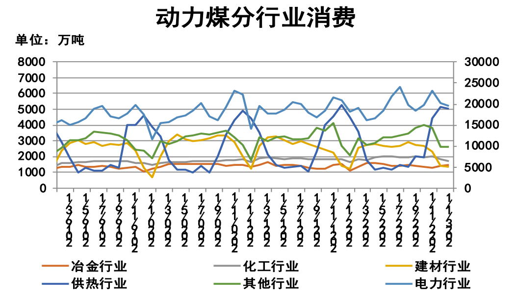
图16、各行业动力煤消费情况
