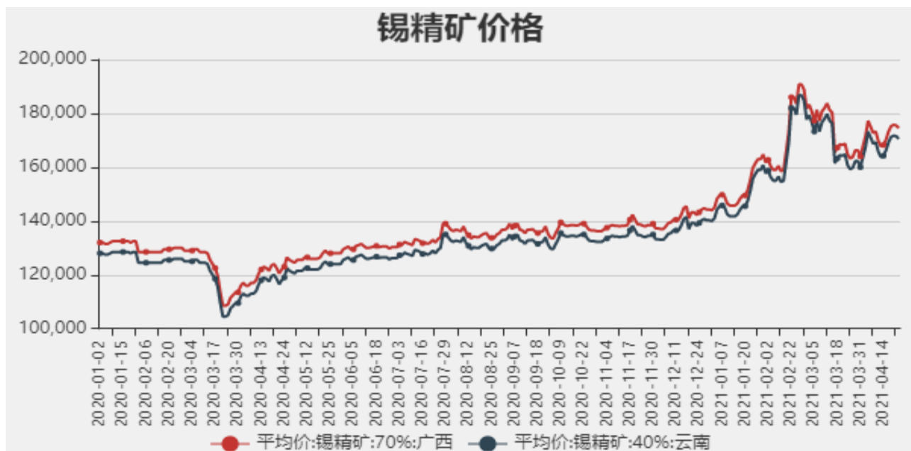
图2：国内锡精矿价格
