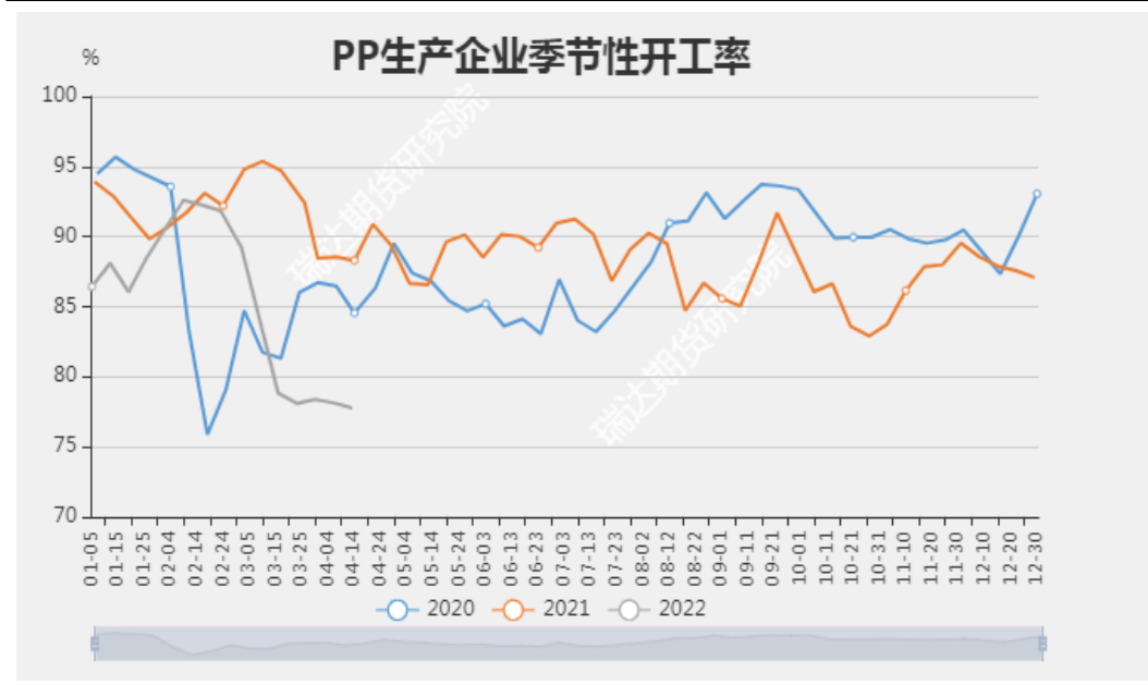
图20、聚丙烯工厂开工率
