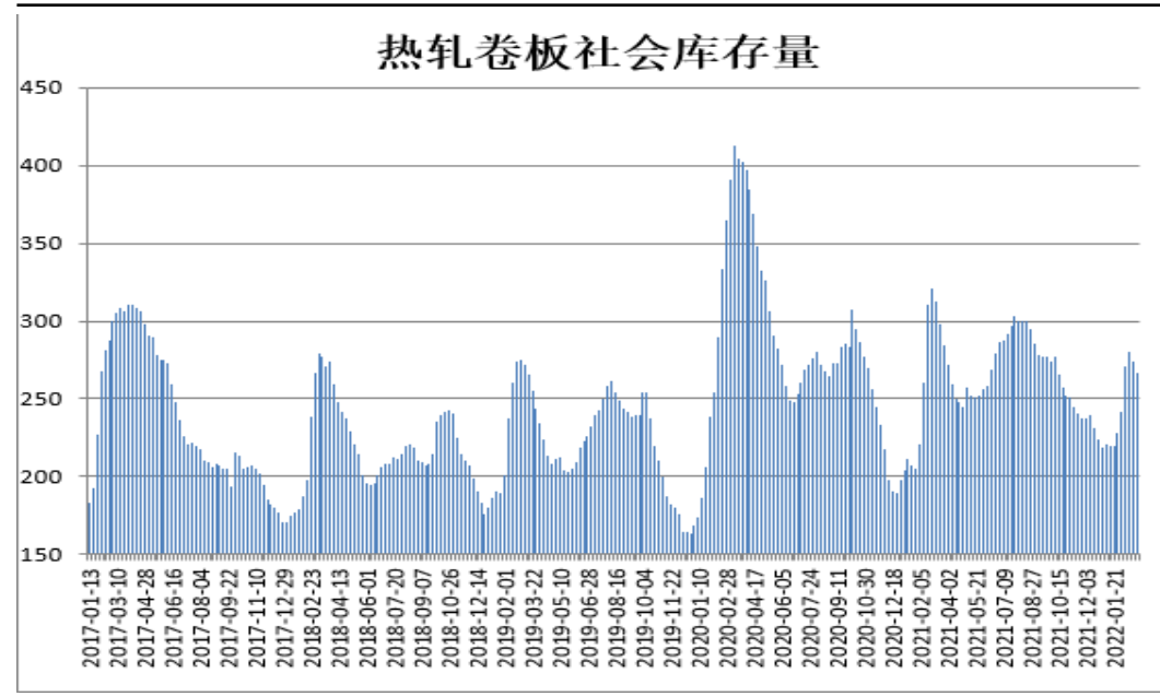
图18、全国33城热轧卷板社会库存
