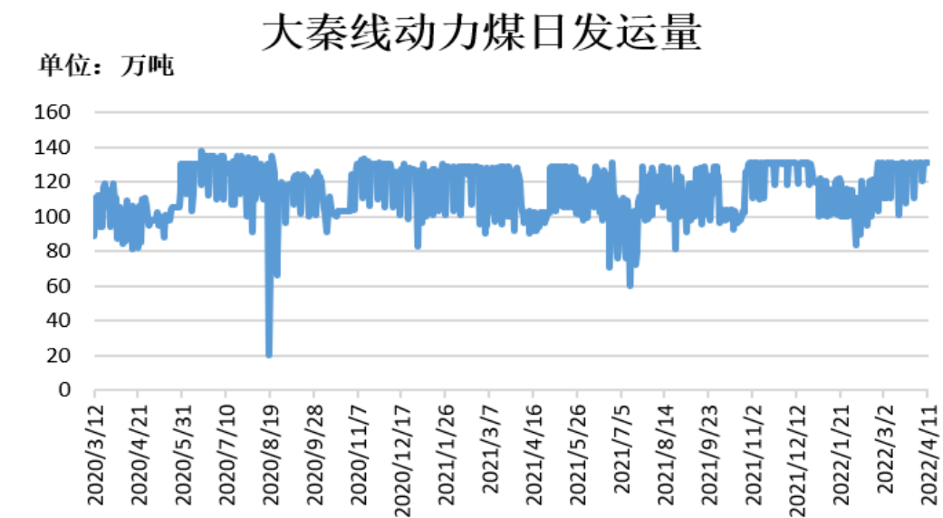
图12、大秦线动力煤日发运量
