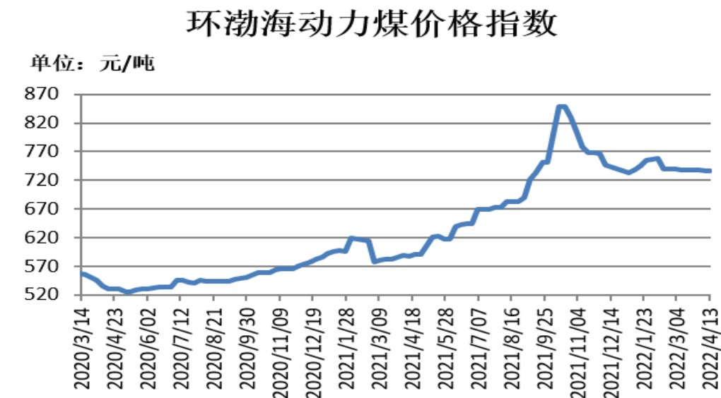
图9、环渤海动力煤价格指数
