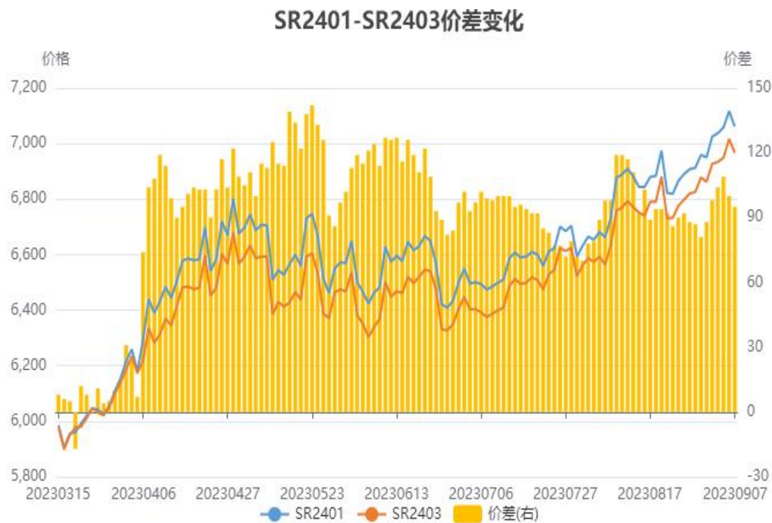
图8、白糖期货1-3价差
