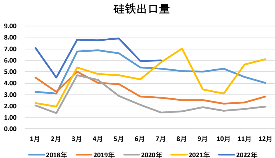
图13、硅铁出口量
