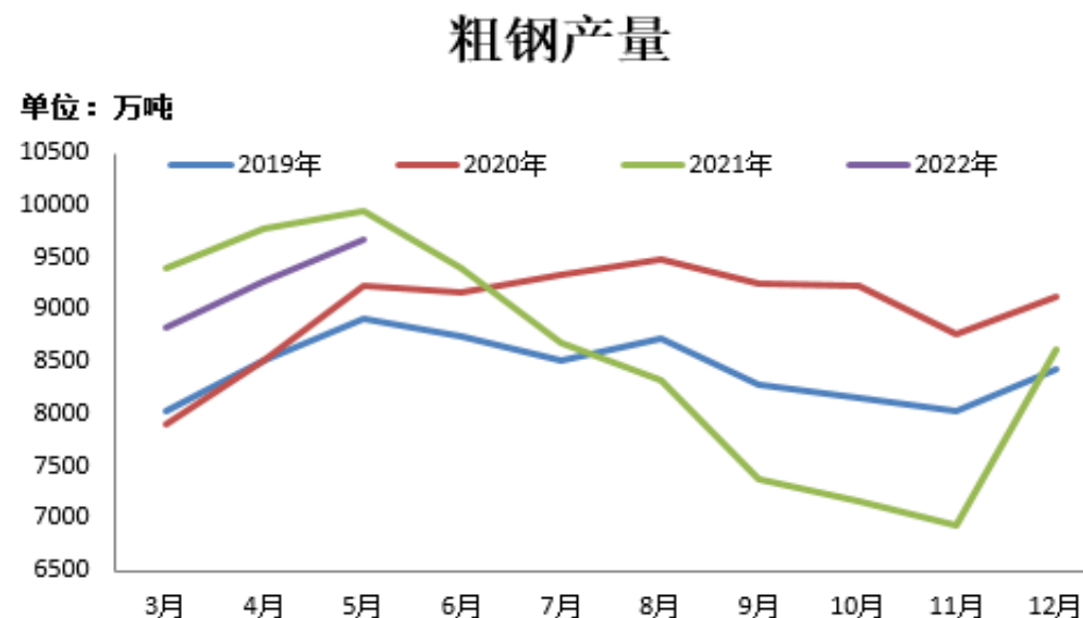
图17、粗钢产量
