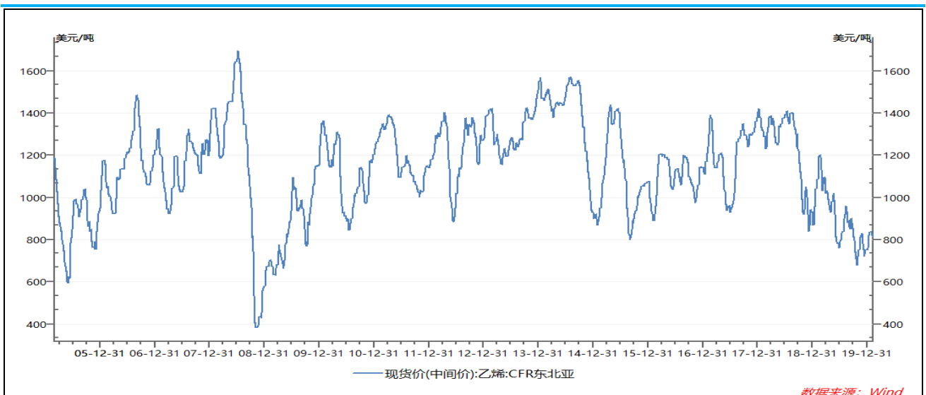
图15 东北亚乙烯现货价
