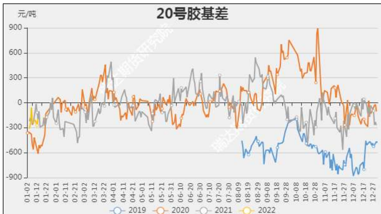
图4 20号胶基差
