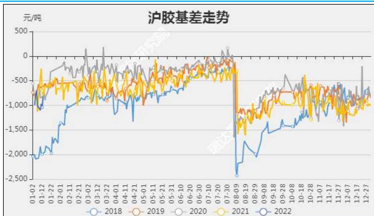
图3 沪胶基差
