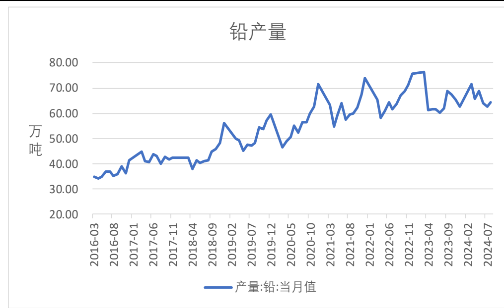
图13、铅产量
