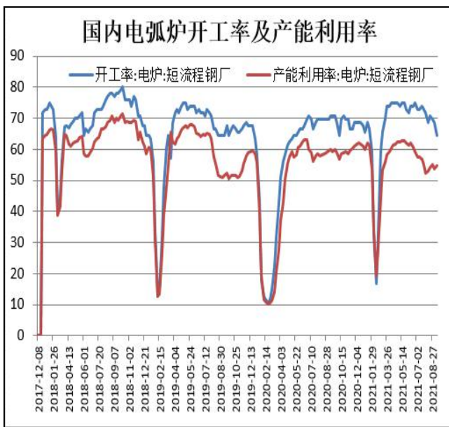
图15：国内电弧炉开工率
