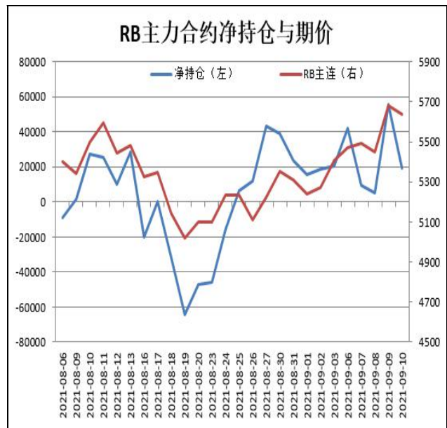
图16：螺纹主力合约前20名净持仓
