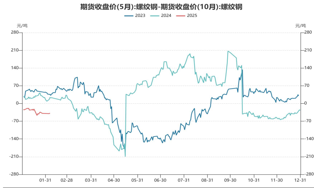
图2、螺纹钢月差
