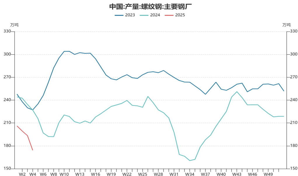
图11、螺纹钢产量
