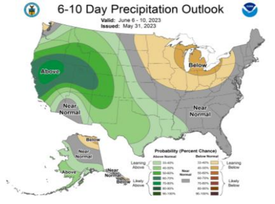
图 0516-0520降水量前瞻
