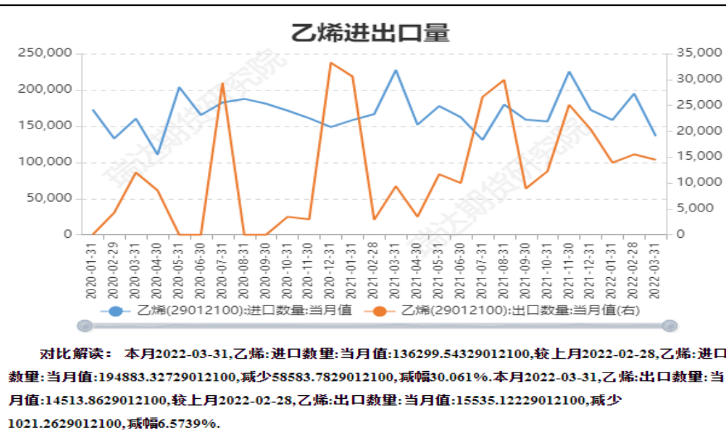
图10、乙烯进出口量
