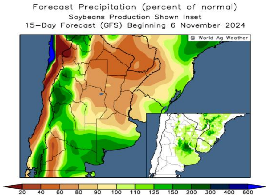
图 阿根廷未来15天降水距平 (%)
