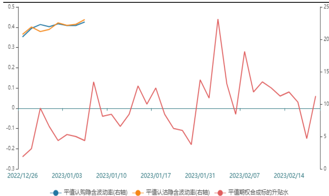
图24、隐含波动率
